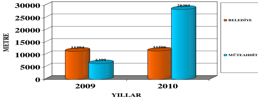
KANALİZASYON DÖŞEME
