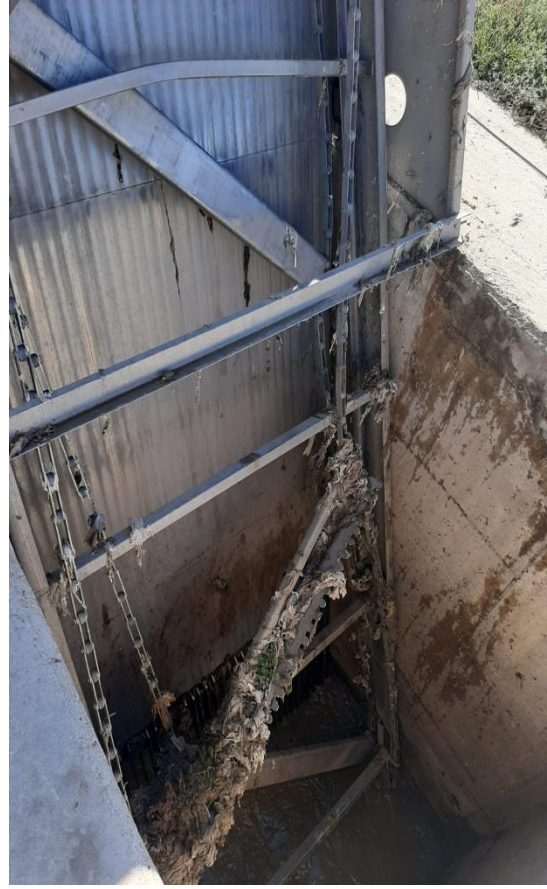
Resim 1: Revizyon Öncesi Arızalı Izgaralar
