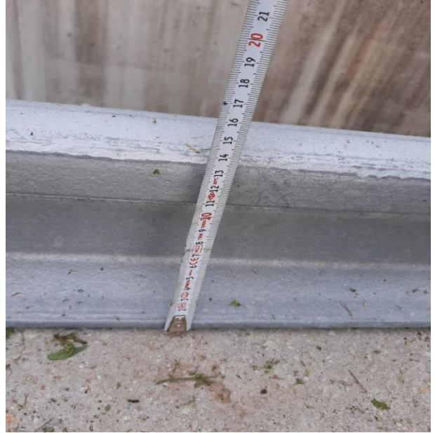
Resim 4: Eski (7,5 cm)-Yeni (13,5 cm) köprü rayları
