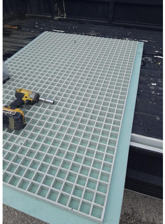
Resim 8: Çürümüş kapaklar yerine CTP kapaklar
