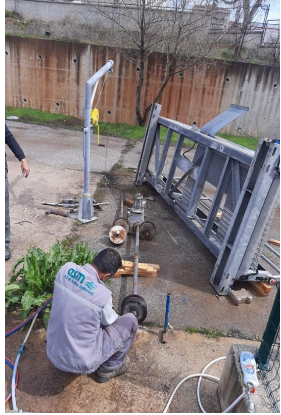
Resim 3: Revizyon Öncesi Arızalı Köprü
